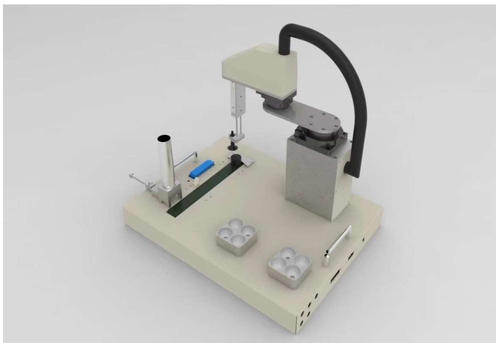
图 3 多功能智能制造竞赛设备机械运动机构图
